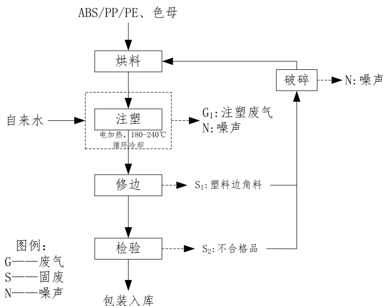
图 2-2 汽车塑料配件生产工艺流程图
