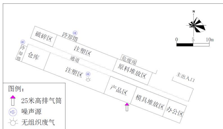
实际车间平面布局
