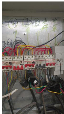
注塑废气处理设施+用电监控
