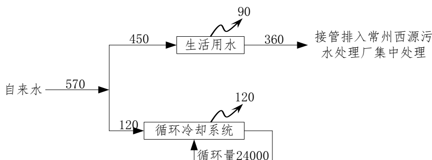
图 2-1 企业水平衡图 (单位 t/a)
